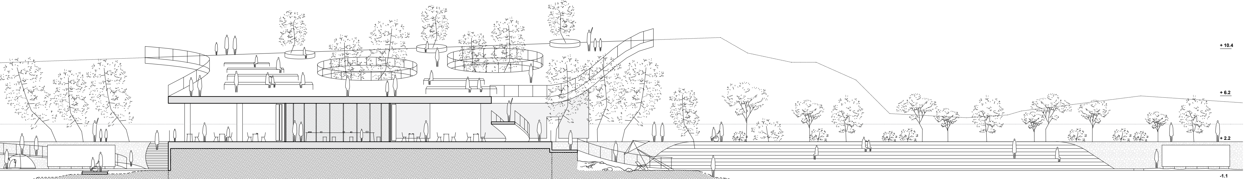
PRESJEK II—II M 1:200
