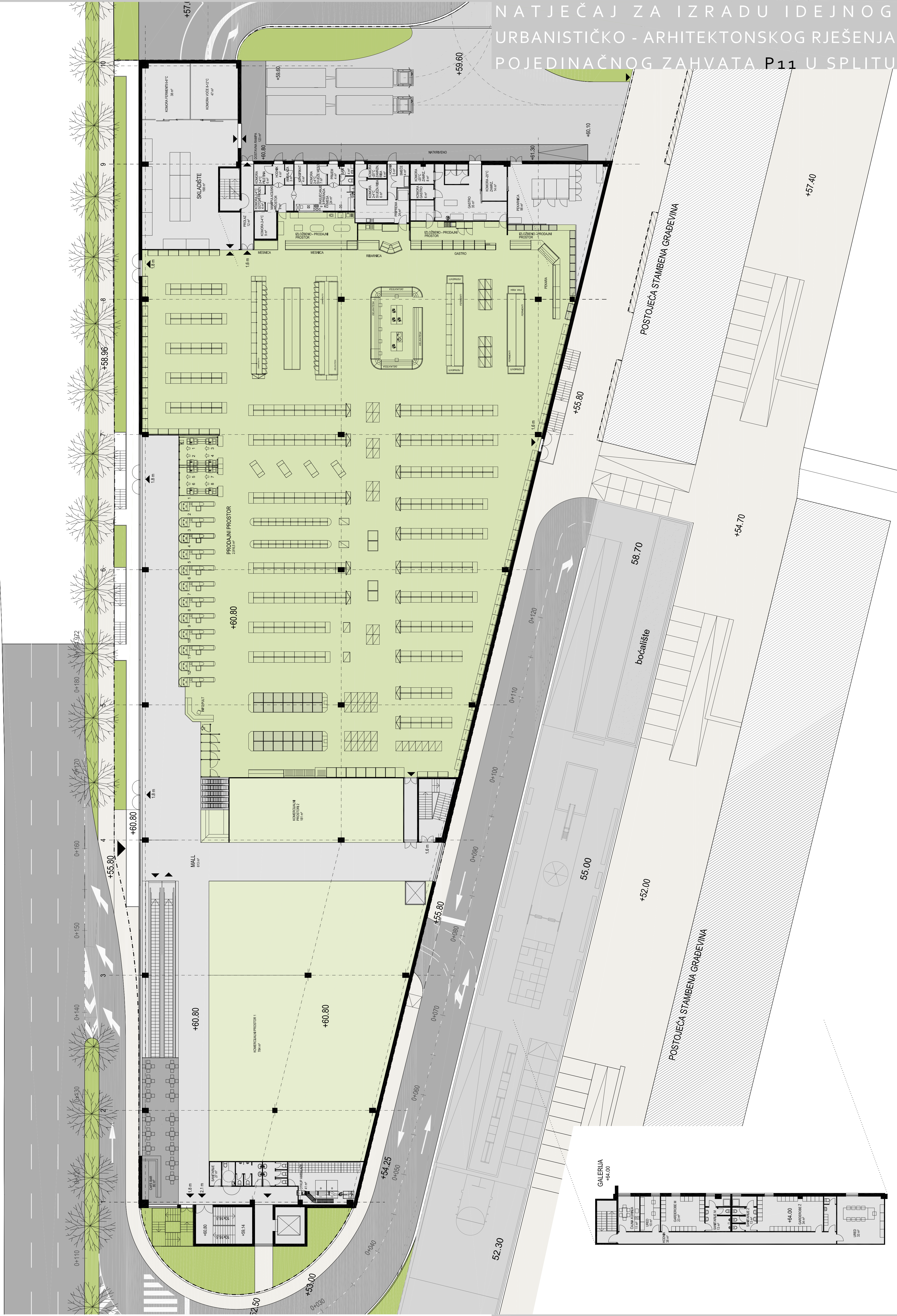
Trgovački centar prizemlje 1:200
